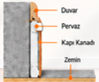
MONTAJ KESİTİ
